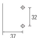
Calço para Dobradiças H88 e H89
