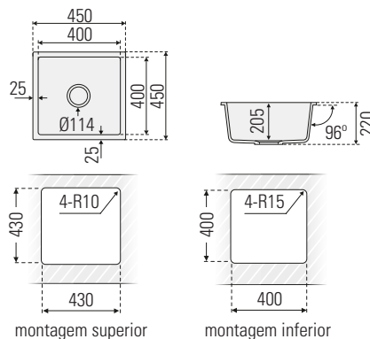
Montagem inferior
