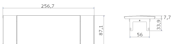
Dimensões da Power Frame Cover Small
