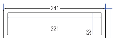
Dimensões da Power Frame Small
