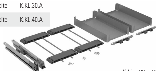
K-Line 30 e 40
