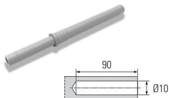
Push-to-Open Tipo 2
