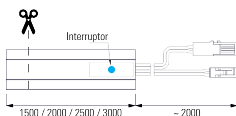
Armadura de embutir com interruptor
