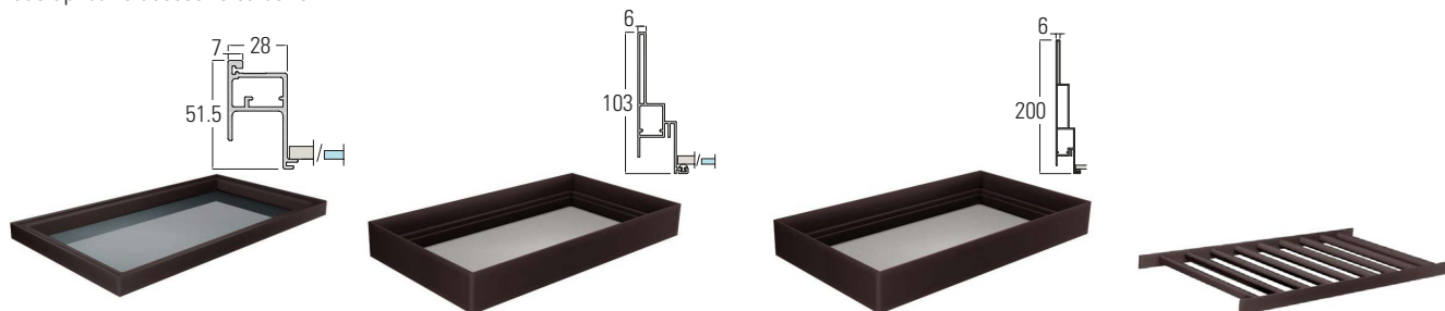
Gaveta com altura de 45 mm.
