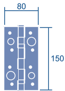
Bisagra antipalanca sin remate canto cuadrado con rodaminetos Referencia: N100AI-R Código: 25921
