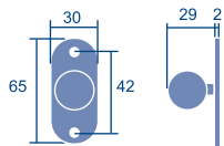
Tirador maletero Referencia: I018 Código: 25946
