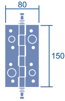
Bisagra antipalanca con remate canto cuadrado Referencia: N115AI Código: 23099
